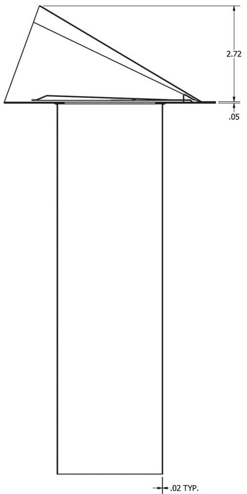
SECTION A-A
