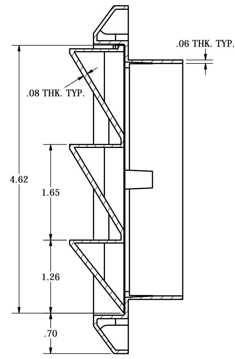
SECTION A-A SCALE 1 : 1
